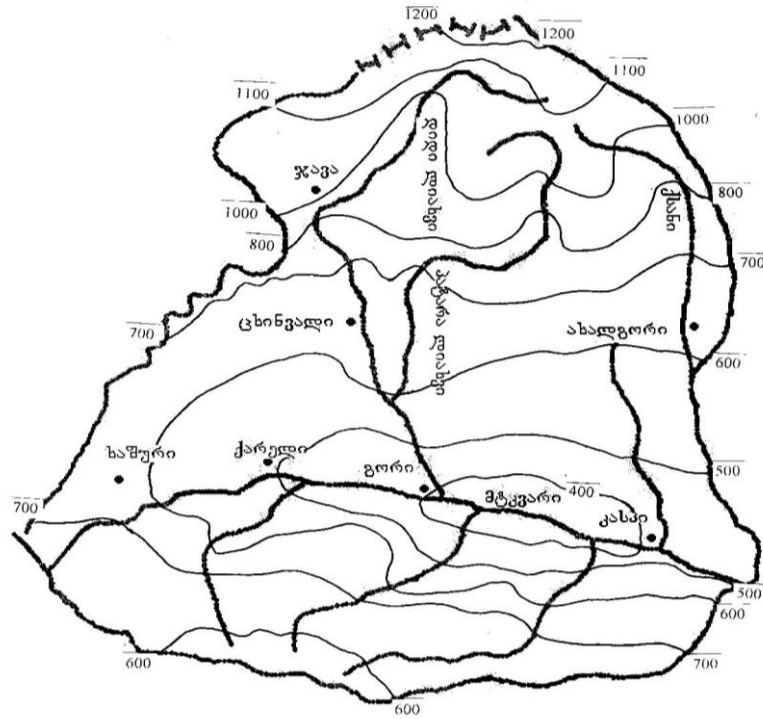
ნახ. 2.3.1. ატმოსფერული ნალექების წლიური ჯამი. მმ.
