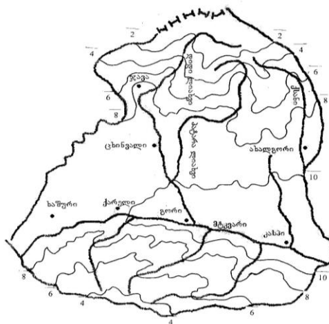
ნახ.2.1.3. ჰაერის საშუალო თვიური ტემპერატურა. აპრილი.
