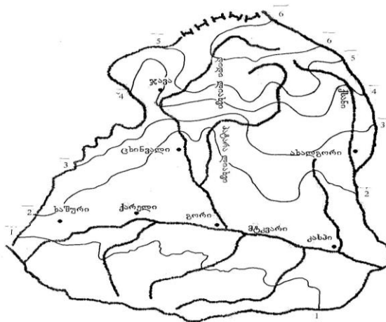
ნახ. 5.2.1. უხვნალექებიან დღეთა რიცხვი იცვლება 10-დან 20 დღემდე.
