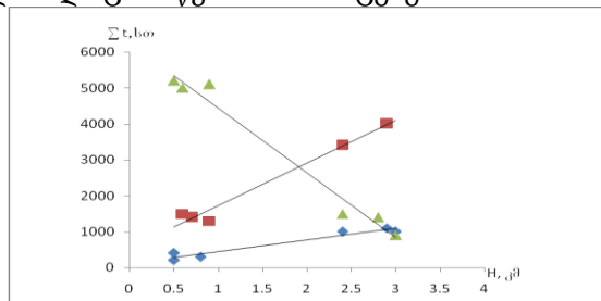
ნახ. 3.3.1 დამოკიდებულება n=f(H) 1- v(0 \dots 2 მ/წმ), 2- v \geq 5 მ/წმ, 3- v \geq 10 მ/წმ
