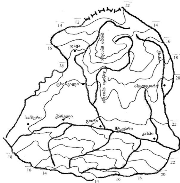
ნახ.2.1.4. ჰაერის საშუალო თვიური ტემპერატურა. ივლისი.
