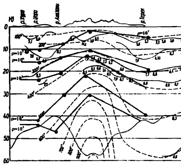
Рис. 1. Зависимость удельного электросопротивления \rho от глубины (температуры)
