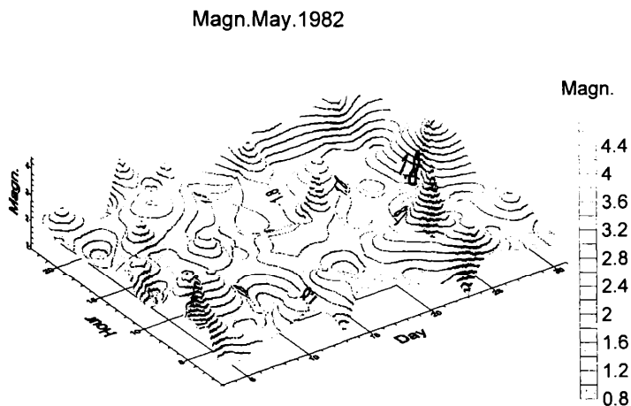
Рис.6 Магнитуда не слабых ( M>2 ) землетрясений в Априле 1982г. от Душети в радиусе 150 км.
