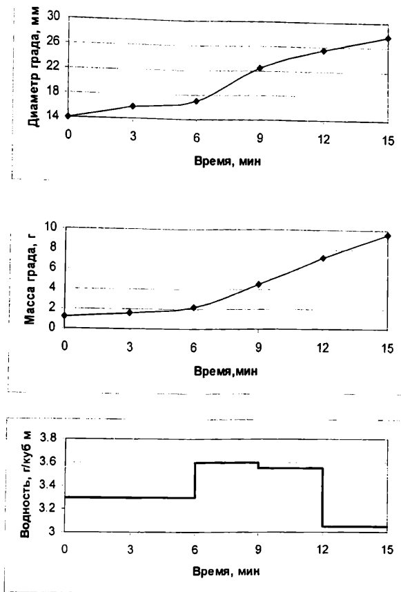
Рис. 2.а Изменение во времени диаметра града (верхний график), его массы (средний график) и водности искусственной облачной среды (нижний график) в опыте № 2. Температура - 18 °С .
