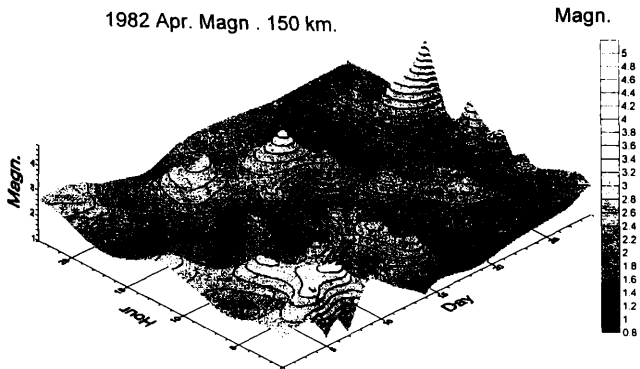
Рис.5 Магнитада неслабых ( M>2 ) землетрясений в Априле 1982г. от Душети в радиусе 150км.
