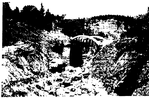
Рис.7. Даниспараулский оползень (Хулойский р-н), сформировавшийся в 2007 г.
