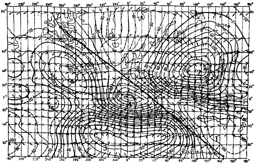
Рис. 2(а,б). Карты вертикальной составляющей геомагнитного поля - изопор вековых геомагнитных вариаций (а [4]) и изодин мировых аномалий (б [5]) для эпохи 1942 г. На картах также приводятся проекции физической земной магнитной оси на поверхности Земли.
