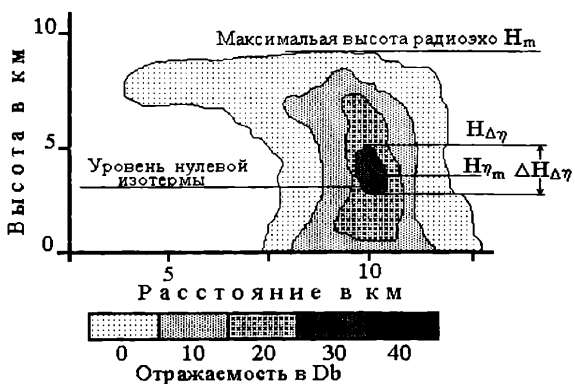
Рис. Схематическое изображение вертикального разреза радиозо одноячейкового конвективного облака ( H_{\Delta\eta} – Верхняя граница зоны повышенной отражаемости; H_{\eta_m} – Высота расположения максимальной радиолокационной отражаемости).
