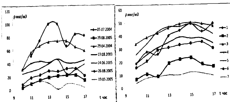
Рис.2. Изменчивость КПО в Академгородке в отдельные дни (слева) и средние значения при разных типах погоды (справа)
