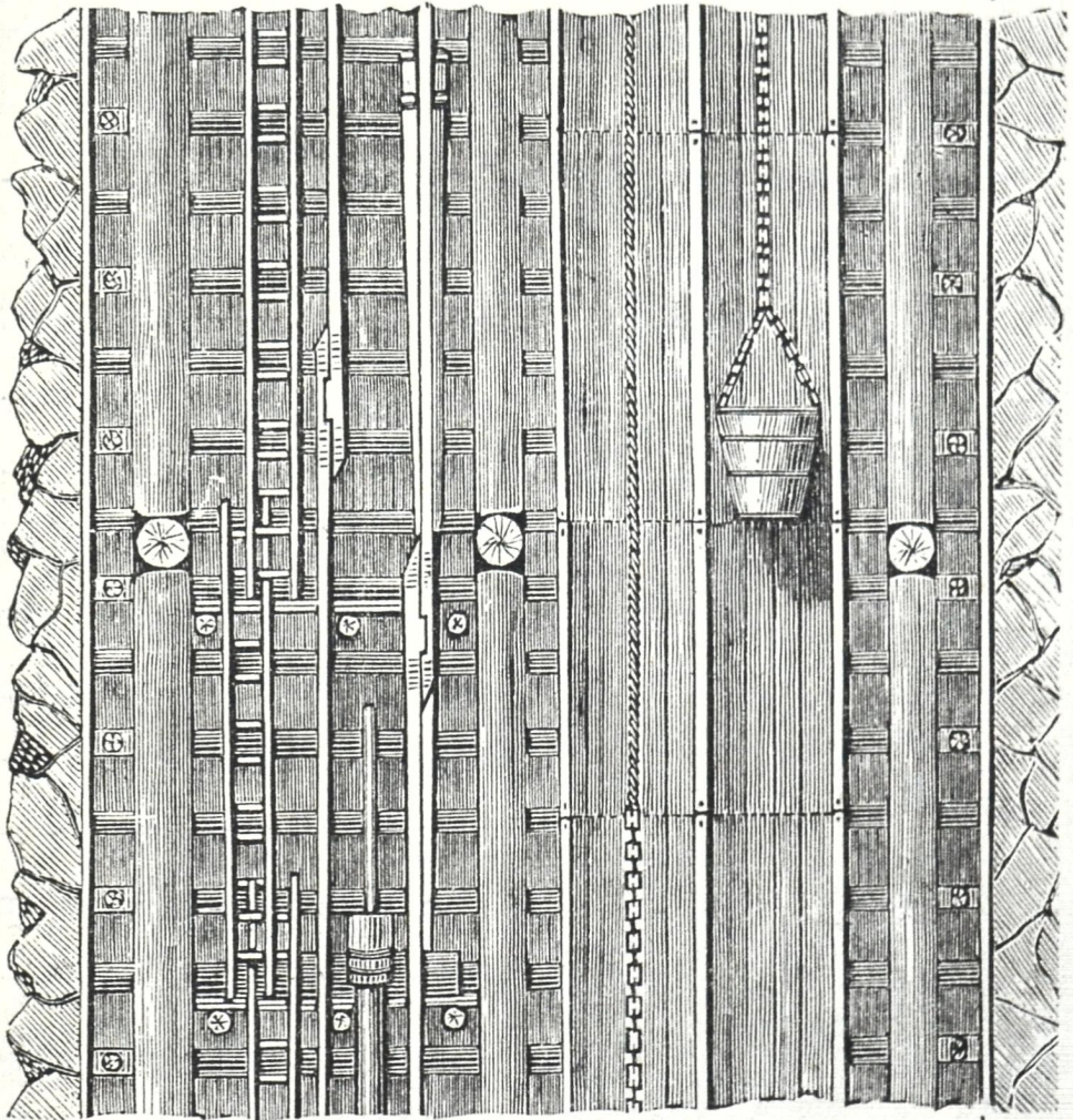
ხის ნაშენობა მადაროებში
