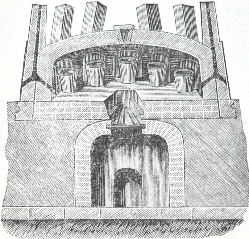
შუმის საკეთებელი ღუმელი
