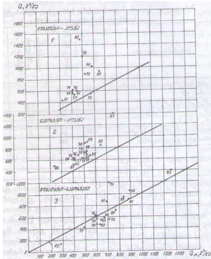
ნახ.1.მდ. რონი _ ს.ალპანას, ნამოხვანისა და გუმათჰესის კვეთე-ბში გავლილი შესატყვისი წყლის მაქსიმალური ხარჯების ურთიერთ დამოკიდებულება (დაკვირვების წლები 1962_1992): 1.გუმათჰესი=f(ალპანა); 2.ნამოხვანი=f(ალპანა); 3.Q გუმათჰესი =f(ნამოხვანი).
