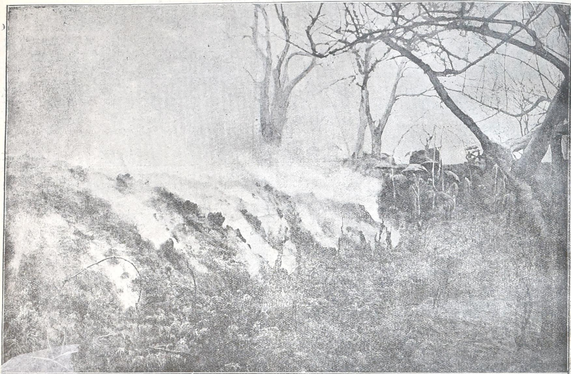
ვეზუვის მთიდან ამოხეთქილი ღვავა დაჟეჟა მთას კალთებზე და წაღეკა ვენ ხეობა, წბადები.
